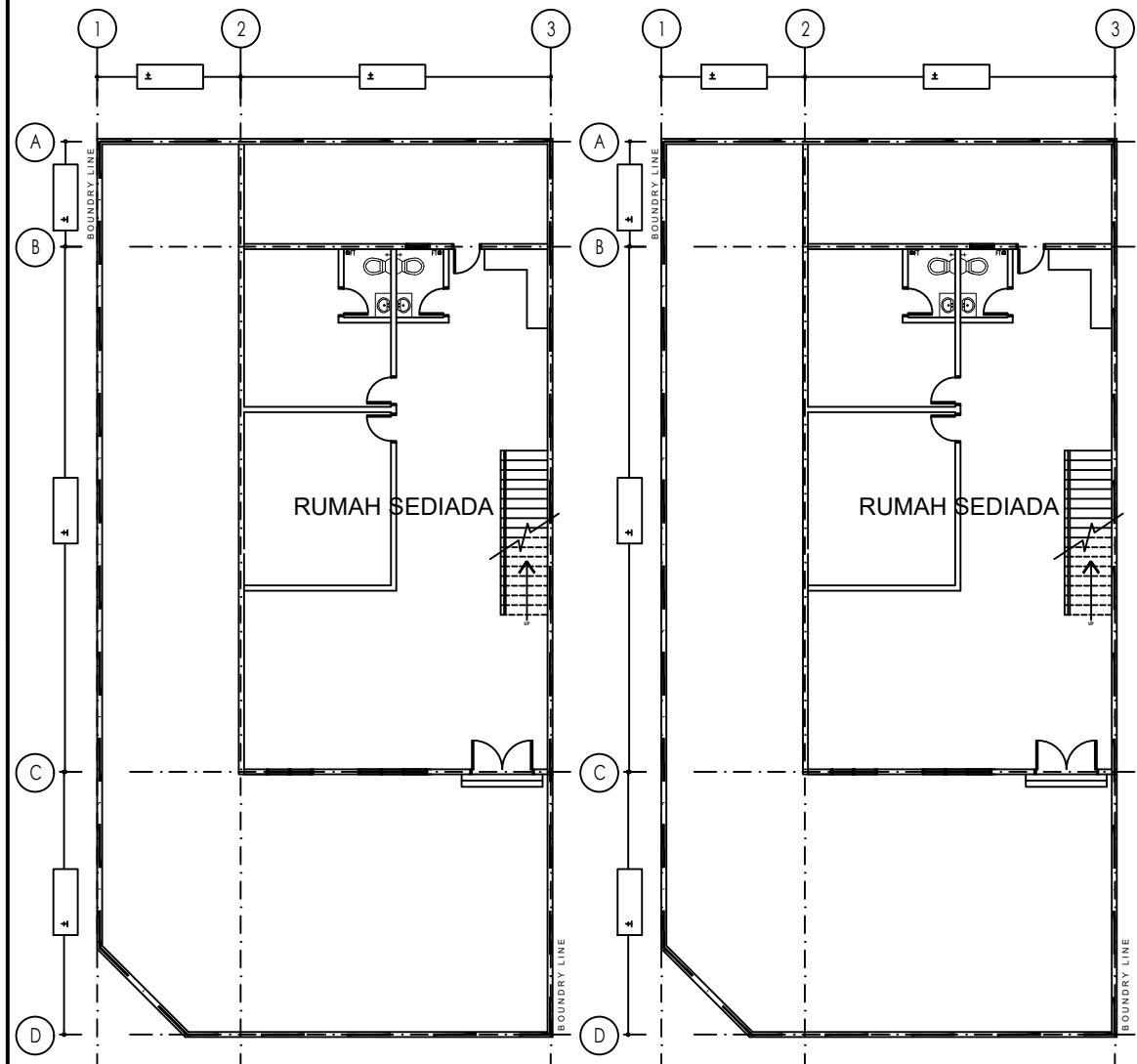
PELAN LANTAI RUMAH TERES 2 TINGKAT
