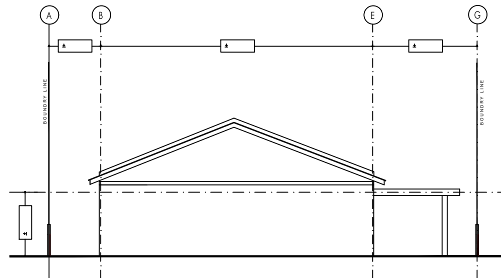
PANDANGAN SISI BINAAN 1 TINGKAT
