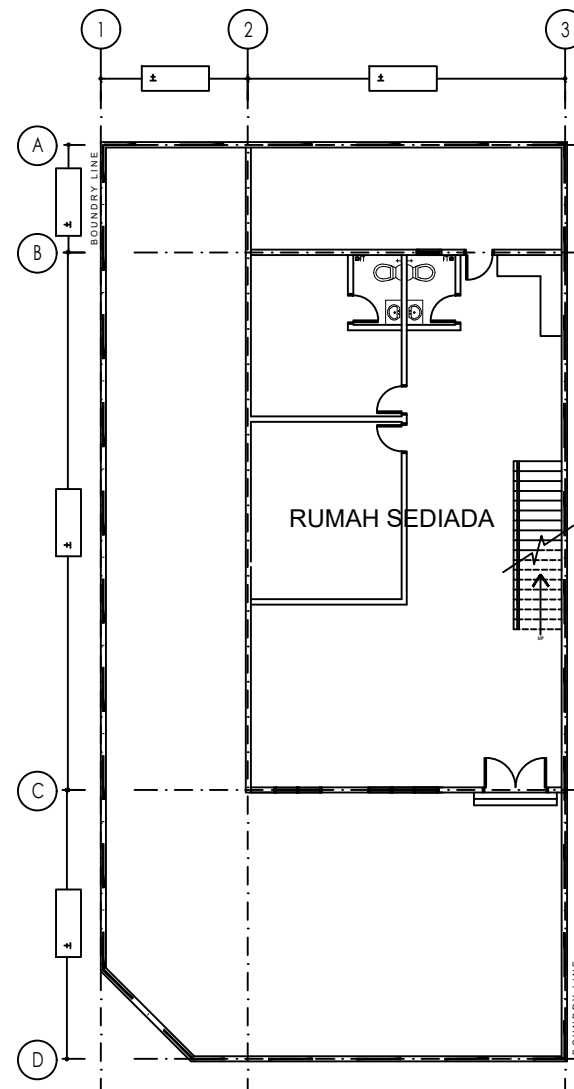
PELAN LANTAI RUMAH TERES 2 TINGKAT
